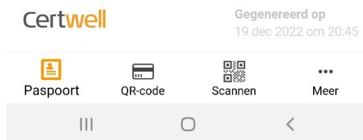
Afb 9.2a Certificaatbeheer
